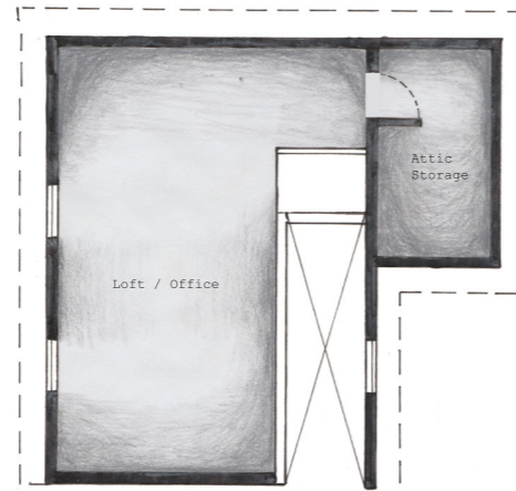
Loft Floorplan - 1/4"=1'
